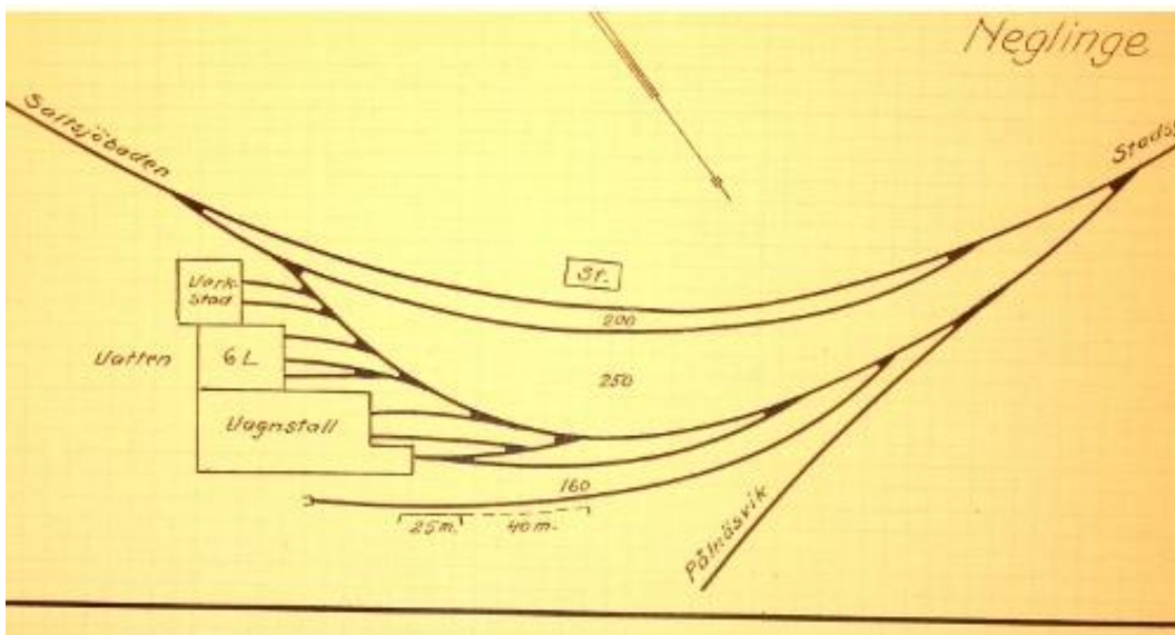
Figur 4. Bangårdsskiss från 1935-talet som visar verkstad, lokstall för sex lok och vagnstall. Saltsjöbanans bangårdar (ckeving.se) och Landgren, Kenneth. Saltsjöbanan. 1993.
